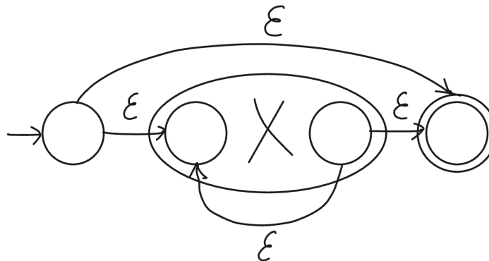
Рис. 3: Итерация X^*
